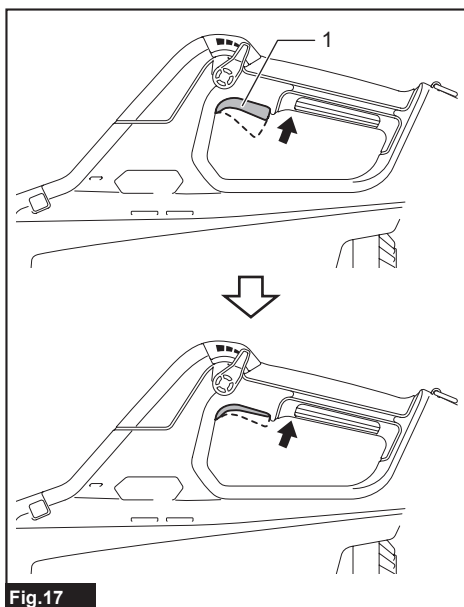
Fig.17 ► 1. Switch trigger
