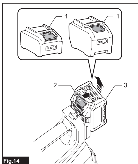
Fig. 14 ► 1. Indicador rojo 2. Botón 3. Cartucho de batería
